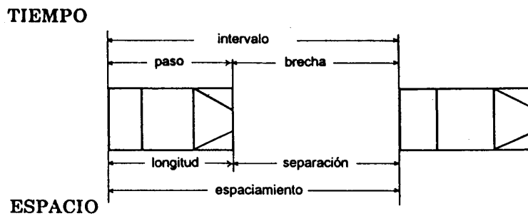
Figura 6-1 Representación gráfica de los parámetros microscópicos de las corrientes vehiculares.
